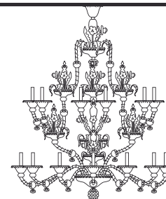
8001/18 H160 Ø135 Lampadario_Chandelier 18 x 60W 230V E14
