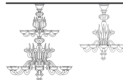
8003/18 H150 Ø120_40 kg Lampadario_Chandelier 18 x 60W 230V E14
