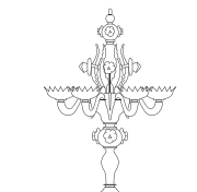
8003/16 H75 Ø 53_7 kg Candelabro_Table candelabrum 6 x 60W 230V E14
