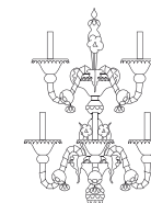
8001/05 H75 Ø60 Applique_wall light 5 x 60W 230V E14
