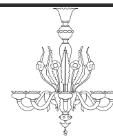
8002/08 H95 Ø 80_15 kg Lampadario_Chandelier 8 x 60W 230V E14
